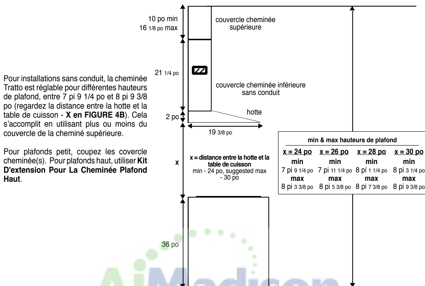
FIGURE 4B INSTALLATIONS SANS CONDUIT
