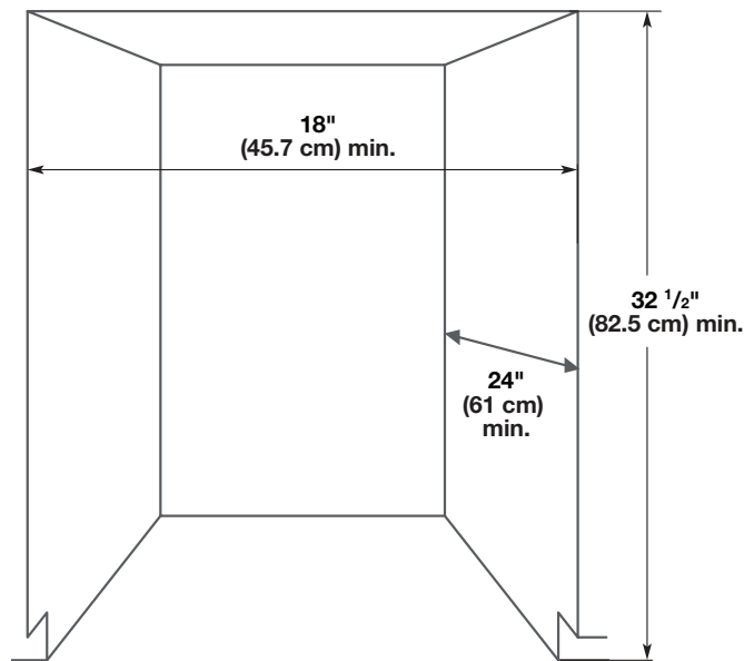
Cutout Dimensions
