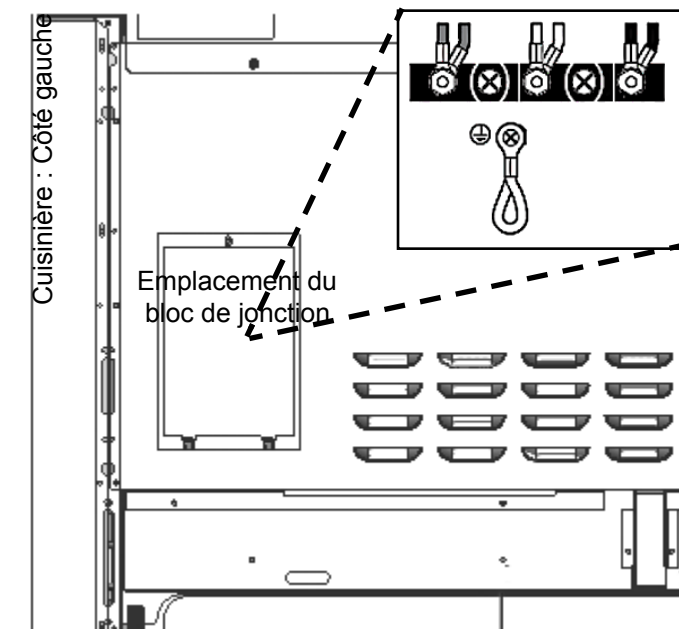
Figure 15: Emplacement du bloc de jonction
