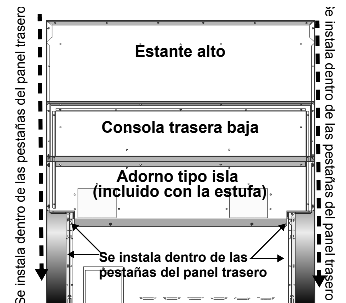
Figura 26: Instalación de la consola trasera baja
