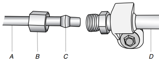
A. Canalisations d'eau du domicile B. Écrou (à acheter) C. Virole (à acheter) D. Tuyau d'eau du réfrigérateur
