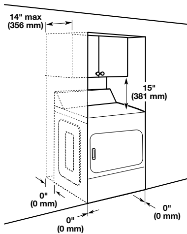
Vue avant, ouverture encastre
