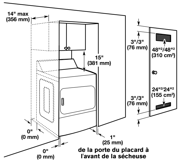
Vue latérale, encasté dans le placard
