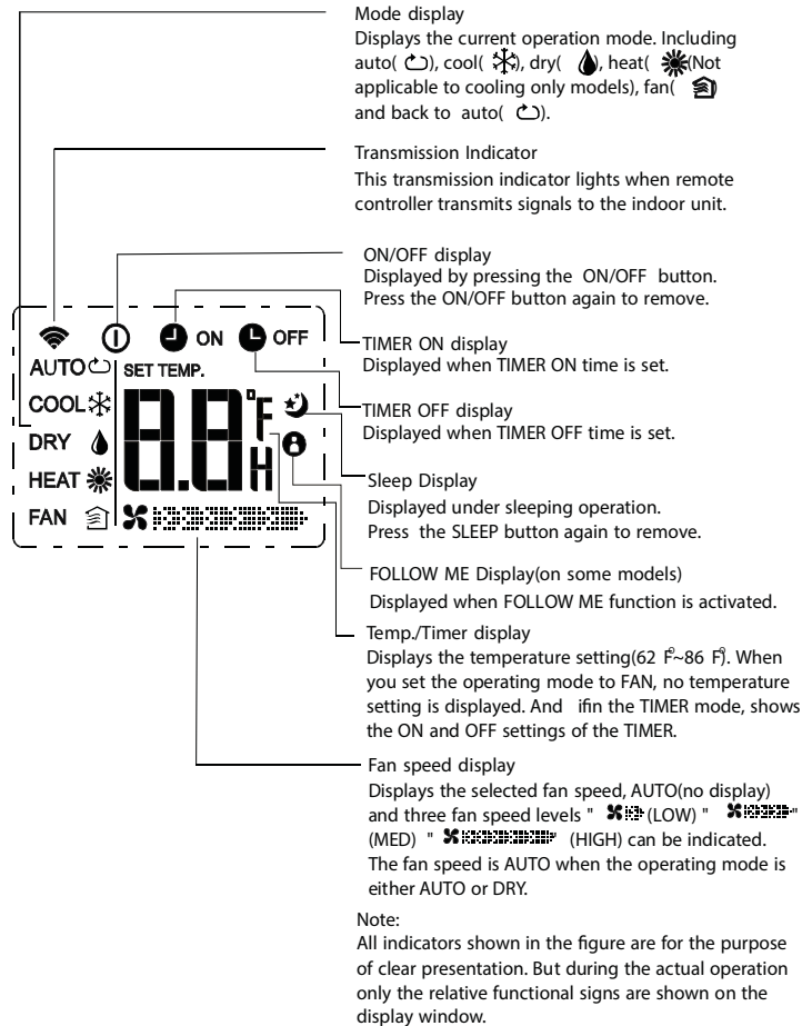
Fig. 4 – Unit Display
