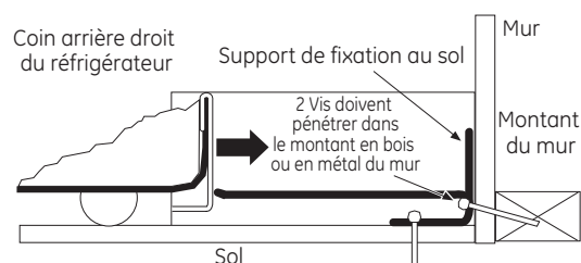
Figure 3 - Fixation au mur et au sol
