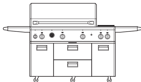
ZGG542NC, barbecue à gaz naturel de 137 cm (54 po) sur chariot avec deux brûleurs latéraux ZGG542LC, barbecue à GPL de 137 cm (54 po) sur chariot avec deux brûleurs latéraux
