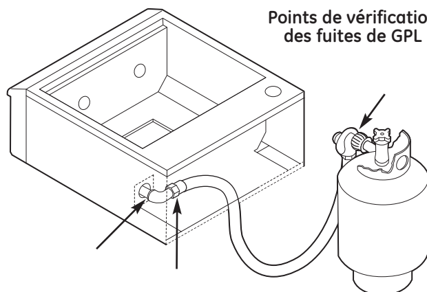
Points de vérification de fuites de GPL avec une table de cuisson
