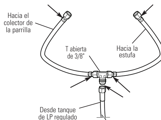
Puntos de prueba de pérdida de gas LP con una estufa
