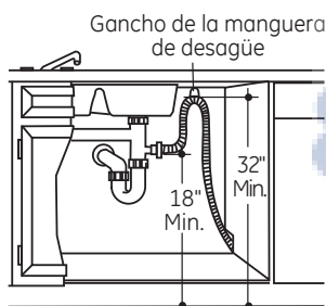
Instalación de la T de desechos
