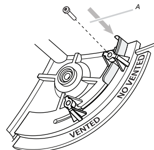
A. Vis de méthode sans ventilation
