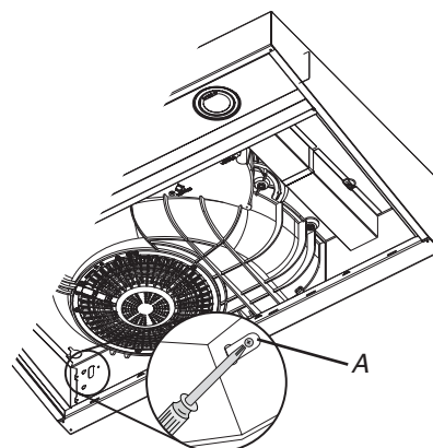
A. Vis no 8-18 x 5/8" (4,2 mm x 16 mm)
