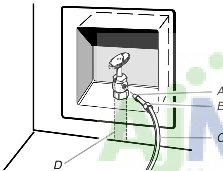
A. Bulbo B. Tuerca C. Tubería de cobre (al refrigerador) D. Línea de suministro doméstica ( \frac{1}{2} " como mínimo)
