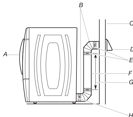
A. Sécheuse B. Coude C. Mur D. Clapet de décharge
