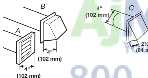
A. Style de clapet à persiennes B. Style de clapet de type boîte C. Style de clapet incliné
