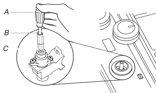
A. Tournevis à tête plate de 3/32" (n° 0 [2 mm]) (la tige doit mesurer au moins 2" [5,1 cm] de long) B. Orifice de la tige du bouton de commande C. Emplacement de la vis de réglage
