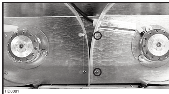
HD0081 Ventilateur double (P8)
