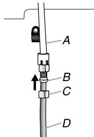
A. Tubería de agua de plástico C. Tuerca de compresión B. Manga D. Tubería de cobre
