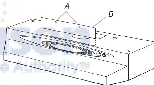
A. Boudoirs de repère B. Plaque du déflecteur
