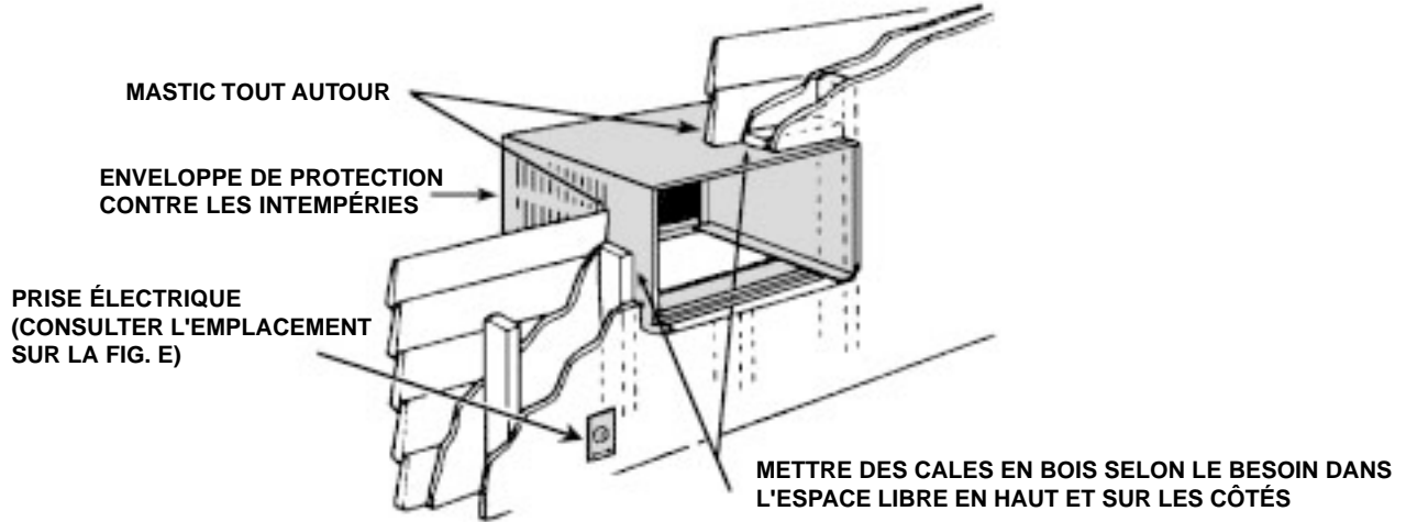
FIGURE C CONSTRUCTIONS AVEC UN CADRE EN BOIS
