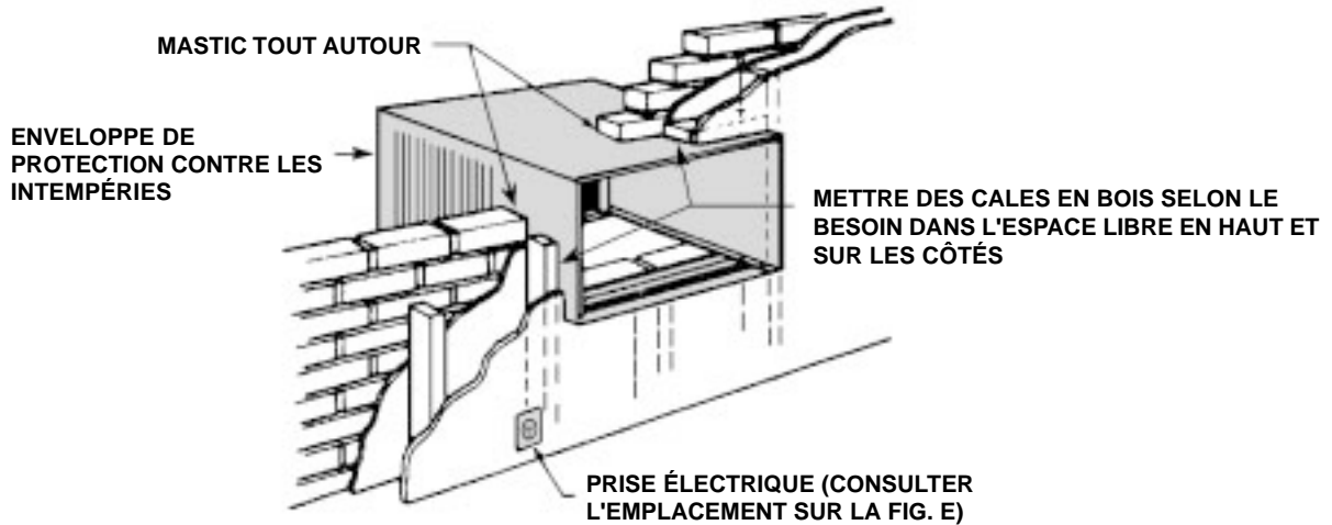
FIGURE D CONSTRUCTION AVEC PAREMENT DE BRIQUE
