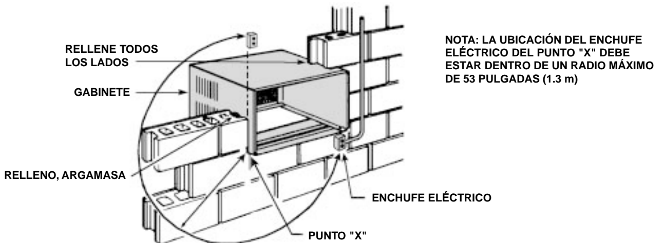
FIGURA E - CONSTRUCCION EN ALBAÑILERÍA SOLIDA
