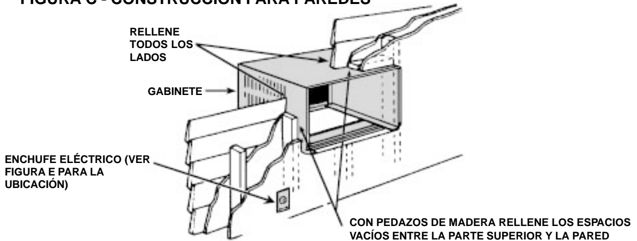
FIGURA C - CONSTRUCCION PARA PAREDES
