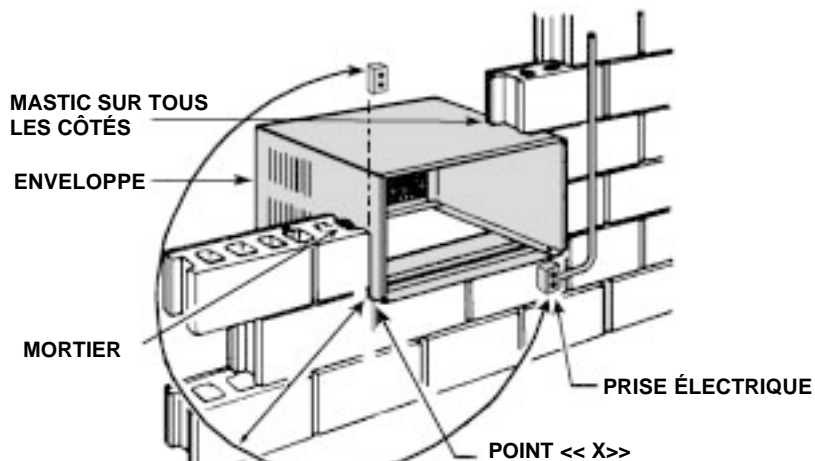
FIGURE E CONSTRUCTION EN MAÇONNERIE SOLIDE
