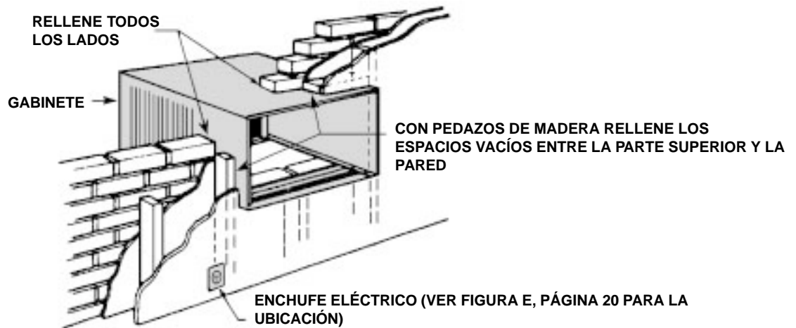
FIGURA D - CONSTRUCCION EN LADRILLO
