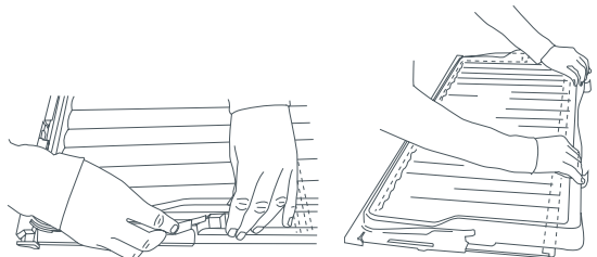
Fig.32 Nettoyage du système de contrôle de l'humidité
