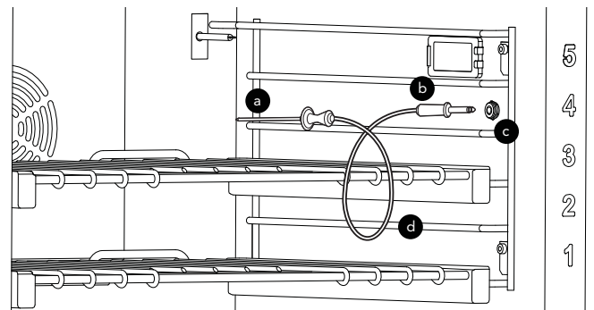
a. Sonda b. Enchufe c. Enchufe de la sonda térmica d. Cable
