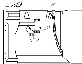
Installation avec un raccord en té d'égout
