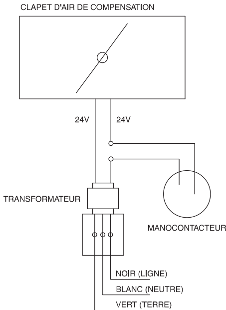
DIAGRAMME DE CÂBLAGE UN CLAPET
