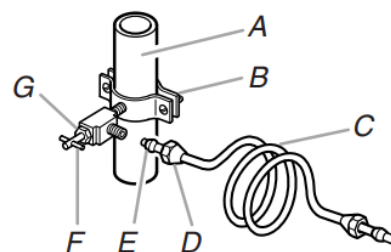
A. Canalisations d'eau froide B. Bride de tuyau C. Tuyau en cuivre ou en polyéthylène réticulé D. Écrou de compression E. Virole de compression F. Robinet d'arrêt G. Écrou de presse-étoupe
