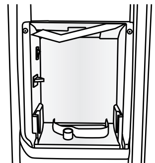
Production de glaçons ON (marche) (bras de commande vers le BAS)
