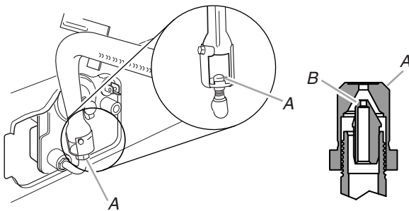
A. Gicleur B. Broche
