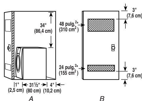
A. Vista lateral - clóset o lugar confinado
