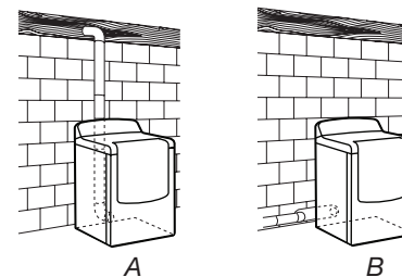
A. Installation de l'évacuation par l'arrière standard en décalage
