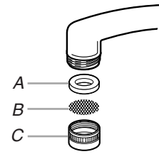
A. Rondelle B. Écran C. Porte-filtre ou aérateur
