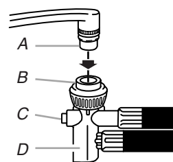
A. Adaptateur pour robinet B. Collet de blocage C. Bouton rouge D. Raccord de tuyau
