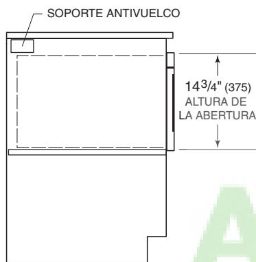
VISTA LATERAL
