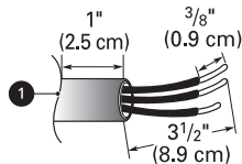
❶ Placa de conexión del cable/conducto
