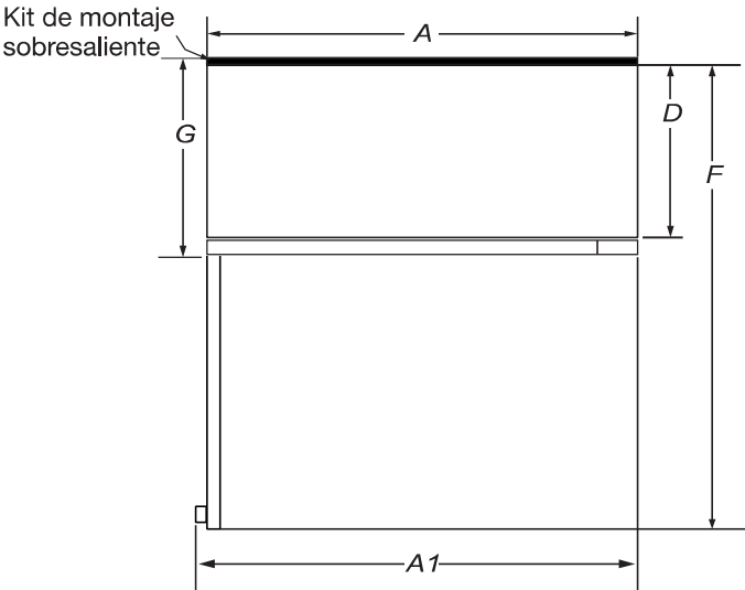
VISTA SUPERIOR
