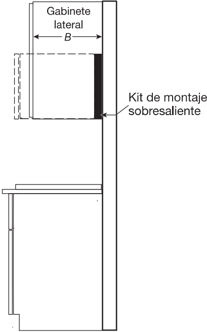
VISTA LATERAL
