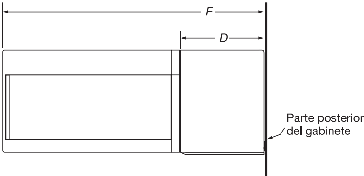
VISTA LATERAL 1
