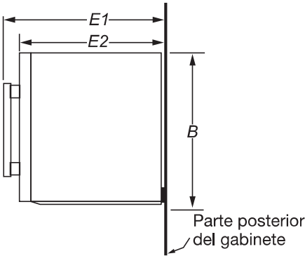
VISTA LATERAL 2
