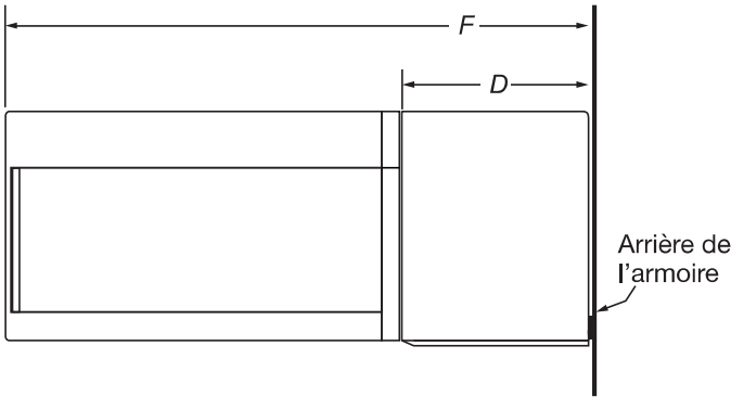
VUE LATÉRALE 1
