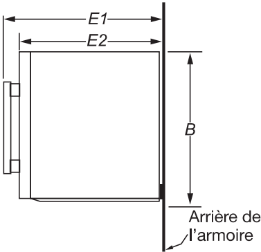
VUE LATÉRALE 2
