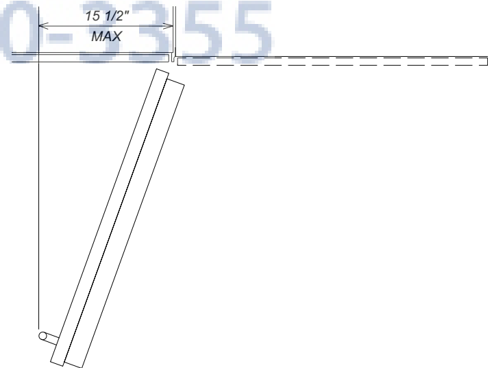
Door Swing
