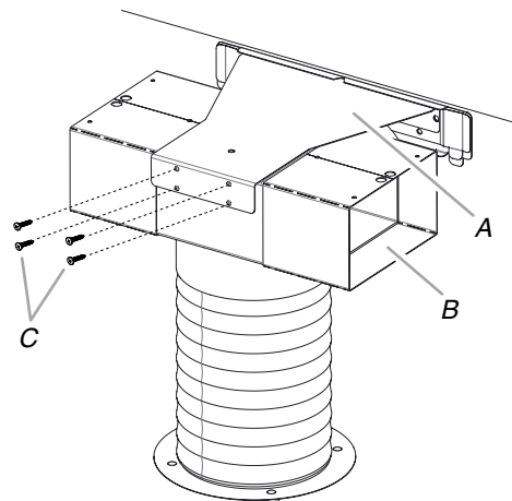
A. Support du déflecteur d'air B. Déflecteur d'air/conduit flexible C. Vis de 3,5 x 9,5 mm (4)
