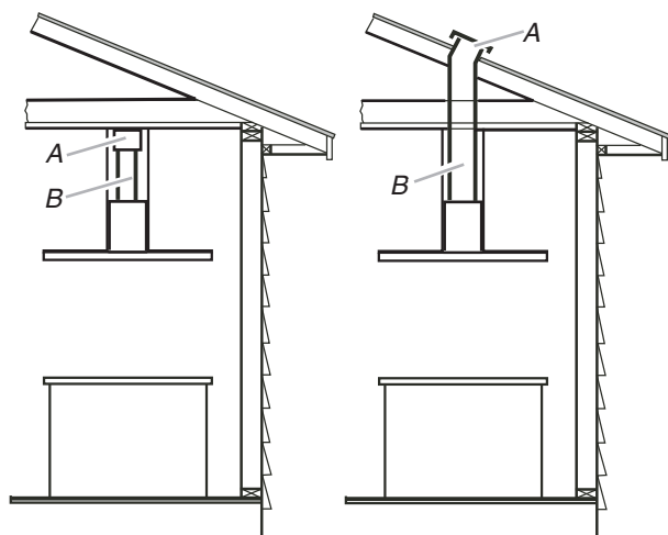
A. Déflecteur
