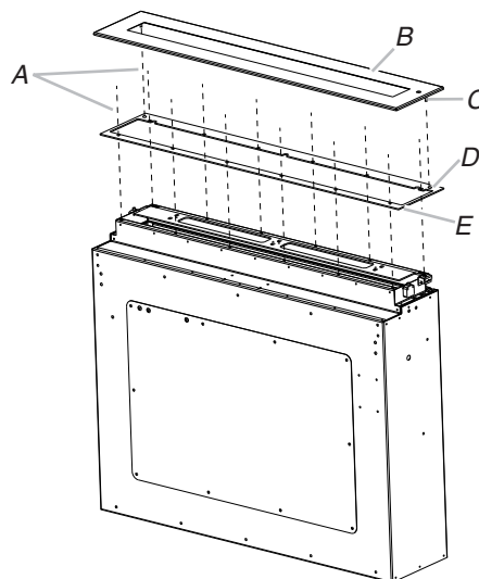
A. 12 vis à tête plate B. Cadre supérieur C. Tiges de guidage du cadre supérieur D. Trou pour les tiges de guidage du cadre supérieur E. Support de cadre supérieur
