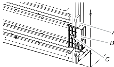
A. Cale d'espacement B. Pied C. Vis n° 8-18 x ¾"
