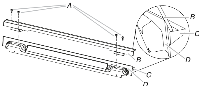
A. Vis n° 8-18 x 1/4" B. Support du déflecteur C. Élément d'évacuation supérieur (fourni avec le four) D. Élément d'évacuation inférieur (fourni avec le four)
