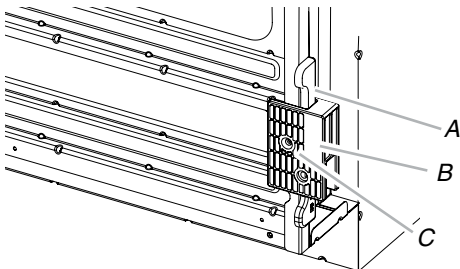
A. Spacer B. Foot C. #8-18 x ¾" screw
