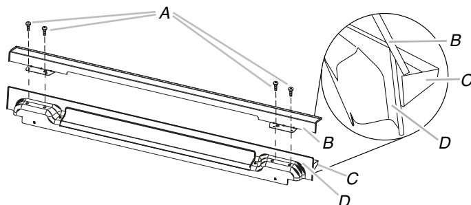
A. Vis n° 8-18 x 1/4" C. Élément d'évacuation supérieur (fourni avec le four) B. Support du déflecteur D. Élément d'évacuation inférieur (fourni avec le four)
