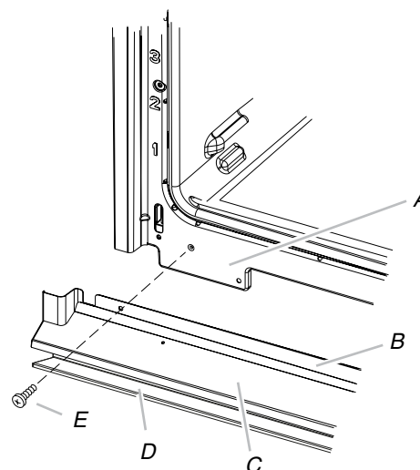
A. Châssis du four D. Support du déflecteur B. Support de l'évent E. Vis n° 8-18 x 3/8"
