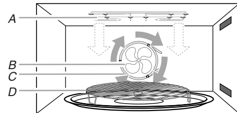
A. Élément de cuisson au gril B. Ventilateur de convection C. Élément de convection D. Grille pour grillades ou grille de cuisson par convection
