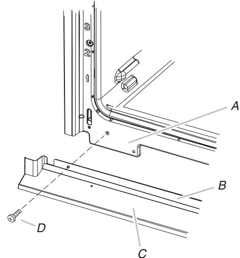
A. Châssis du four B. Support de l'évent
