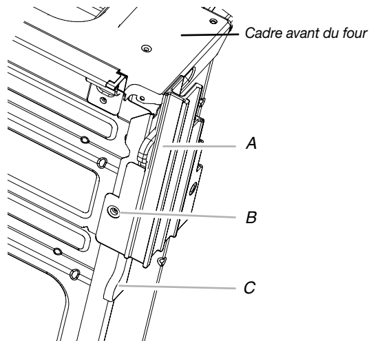
A. Pied avant B. Vis n° 8-18 x ⅜" C. Cale d'espacement
