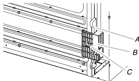
A. Cale d'espacement B. Pied C. Vis n° 8-18 x ⅜"
