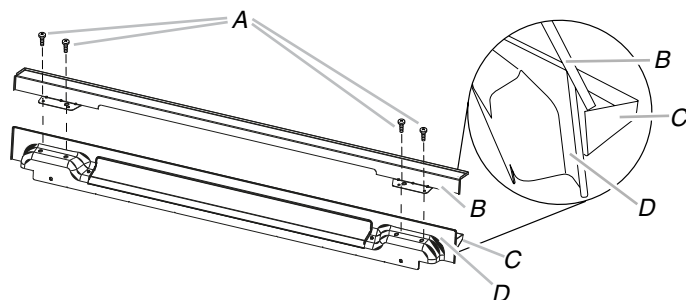
A. Vis n° 8-18 x 1/4" B. Support du déflecteur
