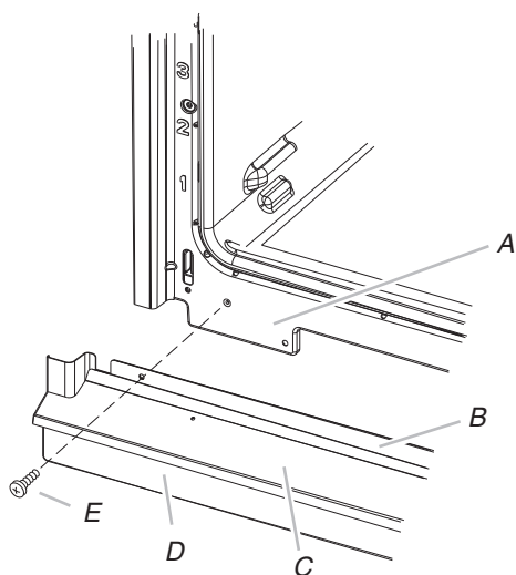
A. Châssis du four D. Garniture de l'évent inférieur B. Support de l'évent E. Vis n° 8-18 x ⅜" C. Évent du four
