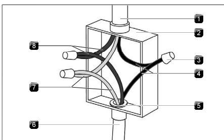
Fig. 11.21 Câble 3 fils
