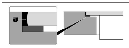
Fig. 11.27 Joint en silicone pour le montage affleurant
