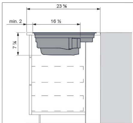
Fig. 11.15 Dimensions de montage pour le dispositif aspirant, profondeur du plan de travail : 23 5 / 8 " [60 cm]
