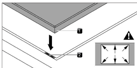
Fig. 11.16 Positionnement des plaques de compensation des hauteurs
