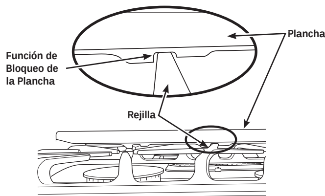
Vista Lateral: Plancha Extraíble y Antiadherente posicionada Correctamente
