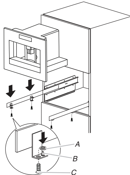
A. Leveling spacers
