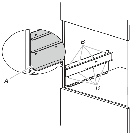
A. Avant de la platine de montage en affleurement avec l'extérieur du cadre du meuble
