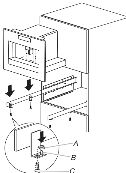
A. Rondelles de nivellement
