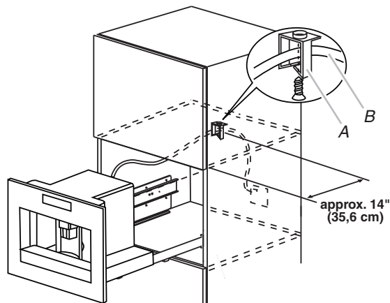
A. Attache du cordon d'alimentation
