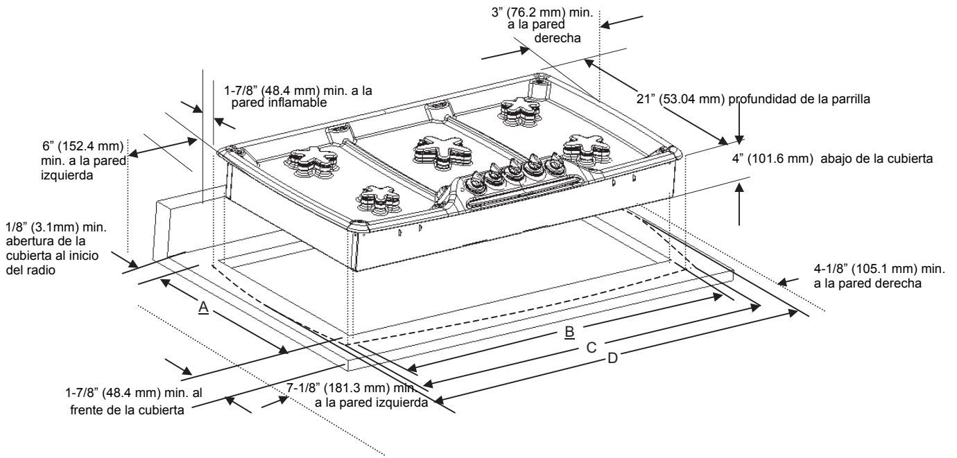
Figura 2 - Dimensiones del recorte
