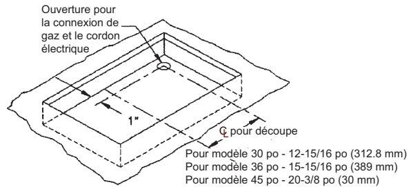
Figure 5 – Zone de la boîte brute
