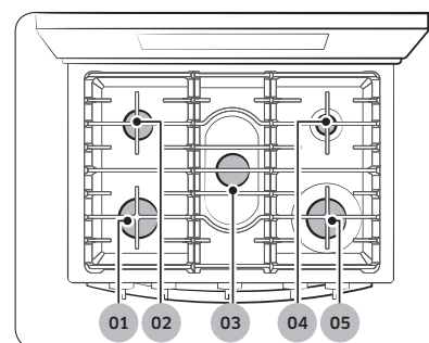
Colocación de los quemadores de la estufa
