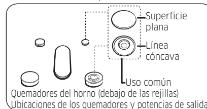
Colocación de los quemadores de la estufa
