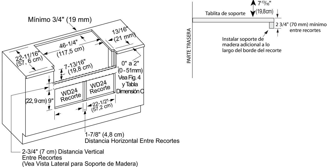
FIG. 8 Instalación de una Parrilla 48" arriba de dos cajones calentadores Thermador lado-a-lado Modelo No. WD24
