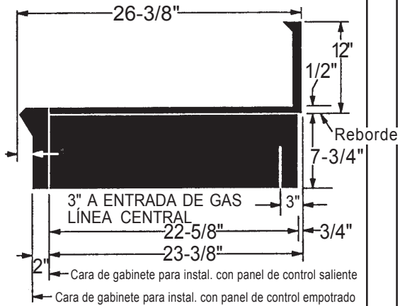
FIG. 5 Vista lateral de la Parrilla
