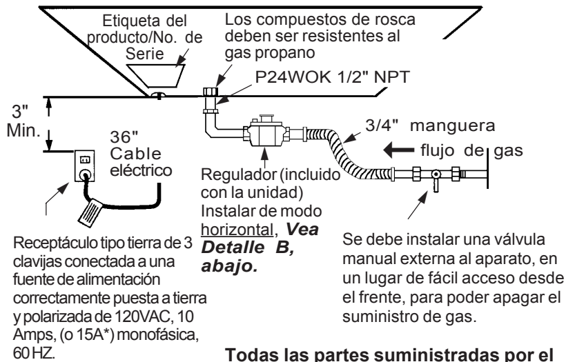
FIG. 9 Frente - Fondo de Unidad, Vea Detalle B, Abajo
