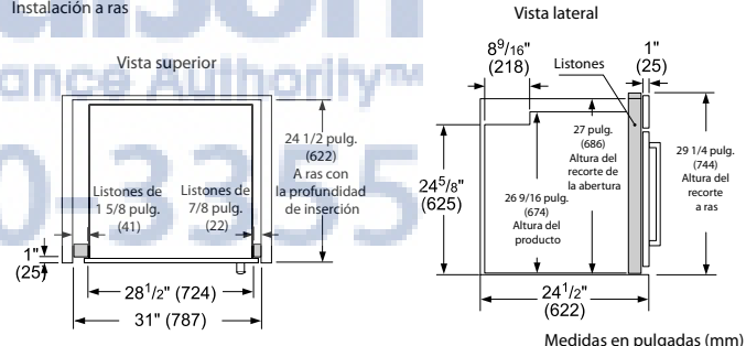
Instalación a ras
