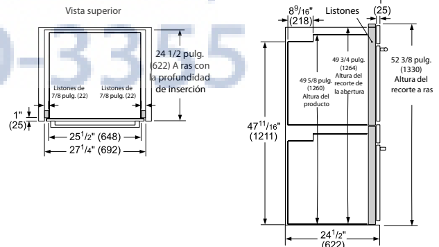
Instalación a ras
