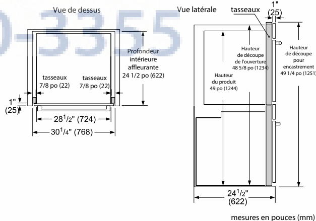
Installation en affleurement
