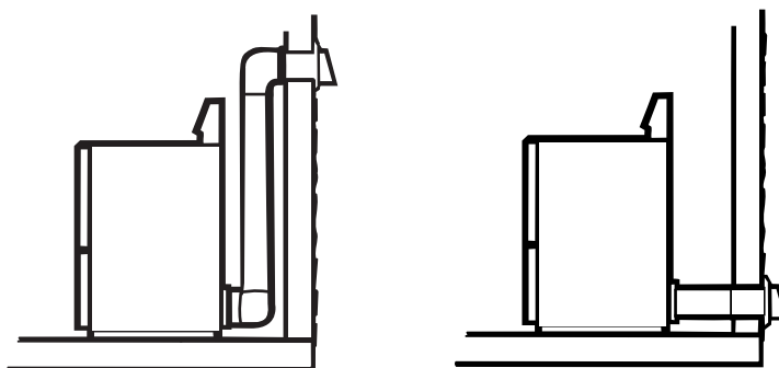
Ventilación correcta
